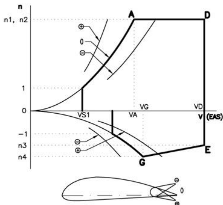
Obr. 1: Obálka obrátů
