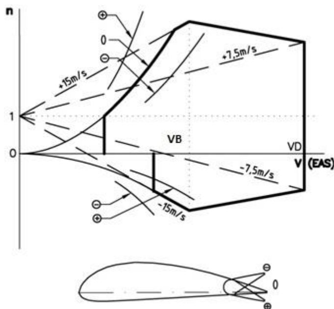
Obr. 2: Poryvová obálka
