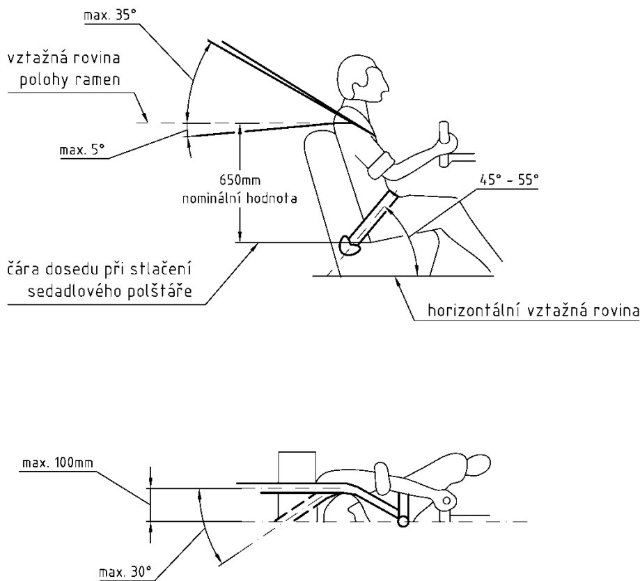
Obr. 3: Doporučená zástavba bezpečnostních pásů
